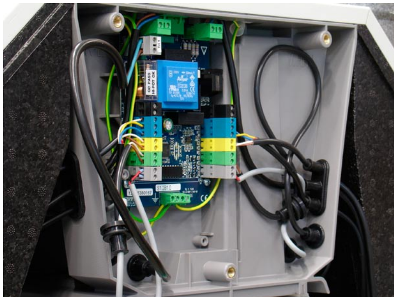
Gekleurde connectoren voorkomen assemblagefouten en zorgen voor servicegemak
